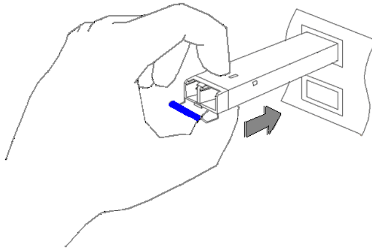
Рисунок 5 – Установка SFP-модуля в верхний разъем SFP
