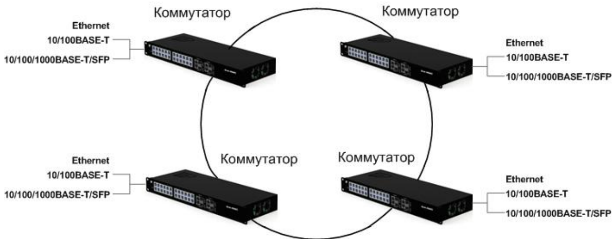
Рисунок 3 – Включение коммутаторов в кольцевую топологию
