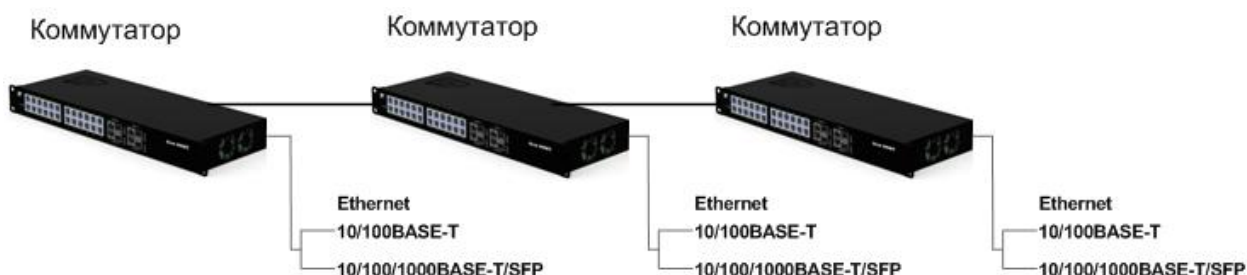
Рисунок 4 – Включение коммутаторов в линейную топологию
