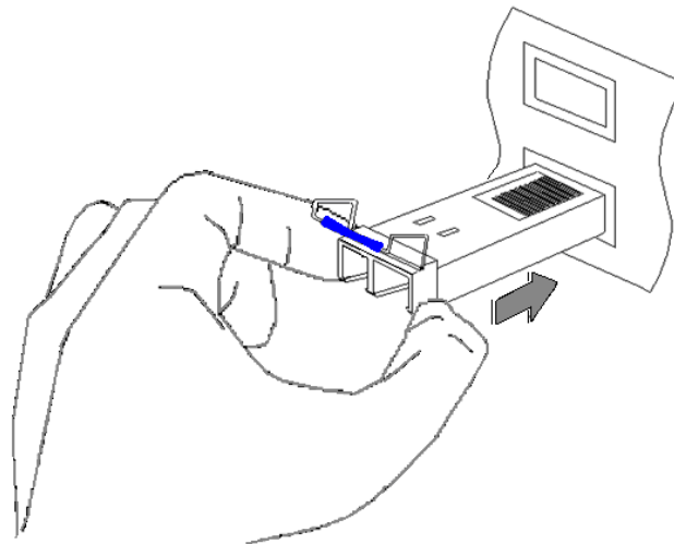
Рисунок 6 – Установка SFP-модуля в нижний разъем SFP
