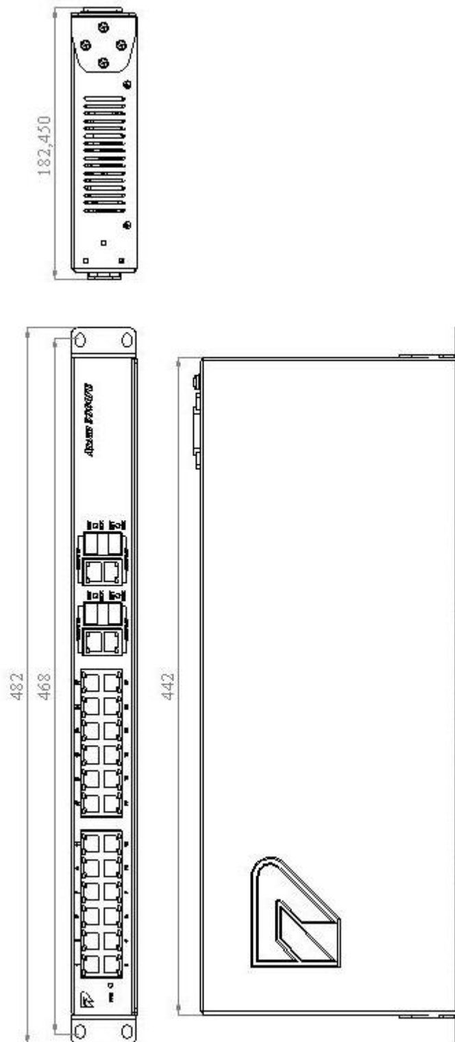
Рисунок А.1 – Габаритные и установочные размеры коммутатора
