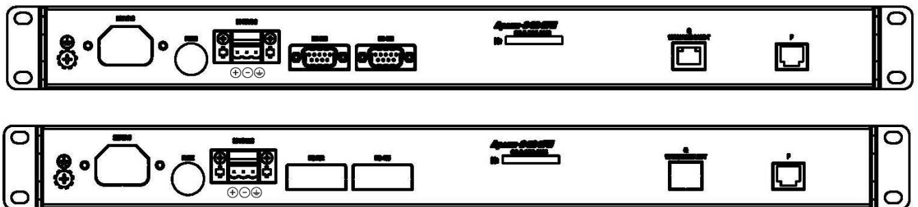
Рисунок Б.3 – Внешний вид задней панели коммутатора в вариантах исполнения с разъемом питания постоянного тока
