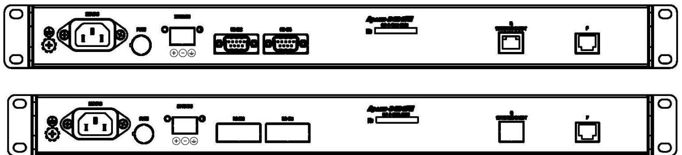
Рисунок Б.2 – Внешний вид задней панели коммутатора в вариантах исполнения с разъемом питания переменного тока
