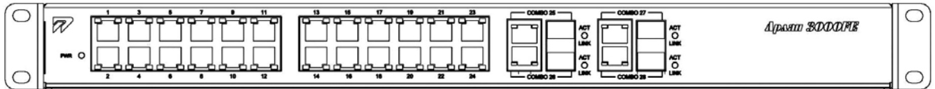
Рисунок Б.1 – Внешний вид лицевой панели коммутатора
