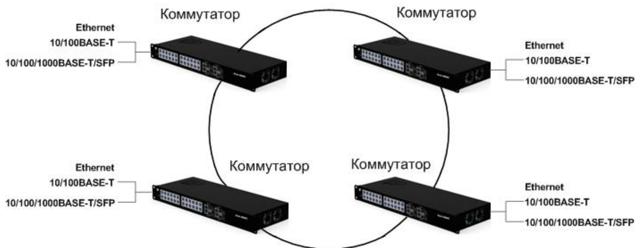
Рисунок 2 – Включение коммутаторов в кольцевую топологию
