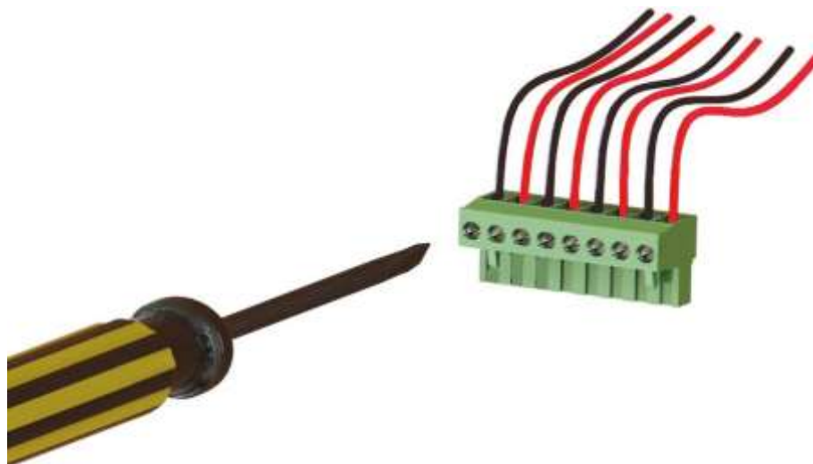
Рисунок 7 – Подключение проводов к ответной части разъема «сухие контакты»
