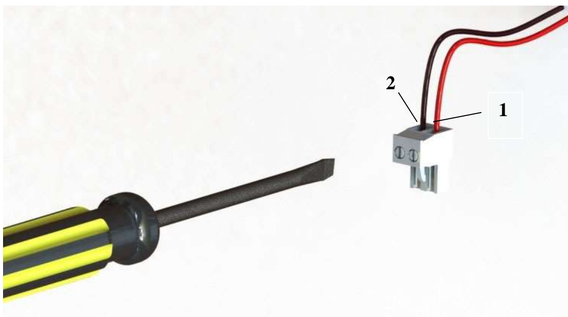
1 – положительный провод (красный); 2 – отрицательный провод (черный)
