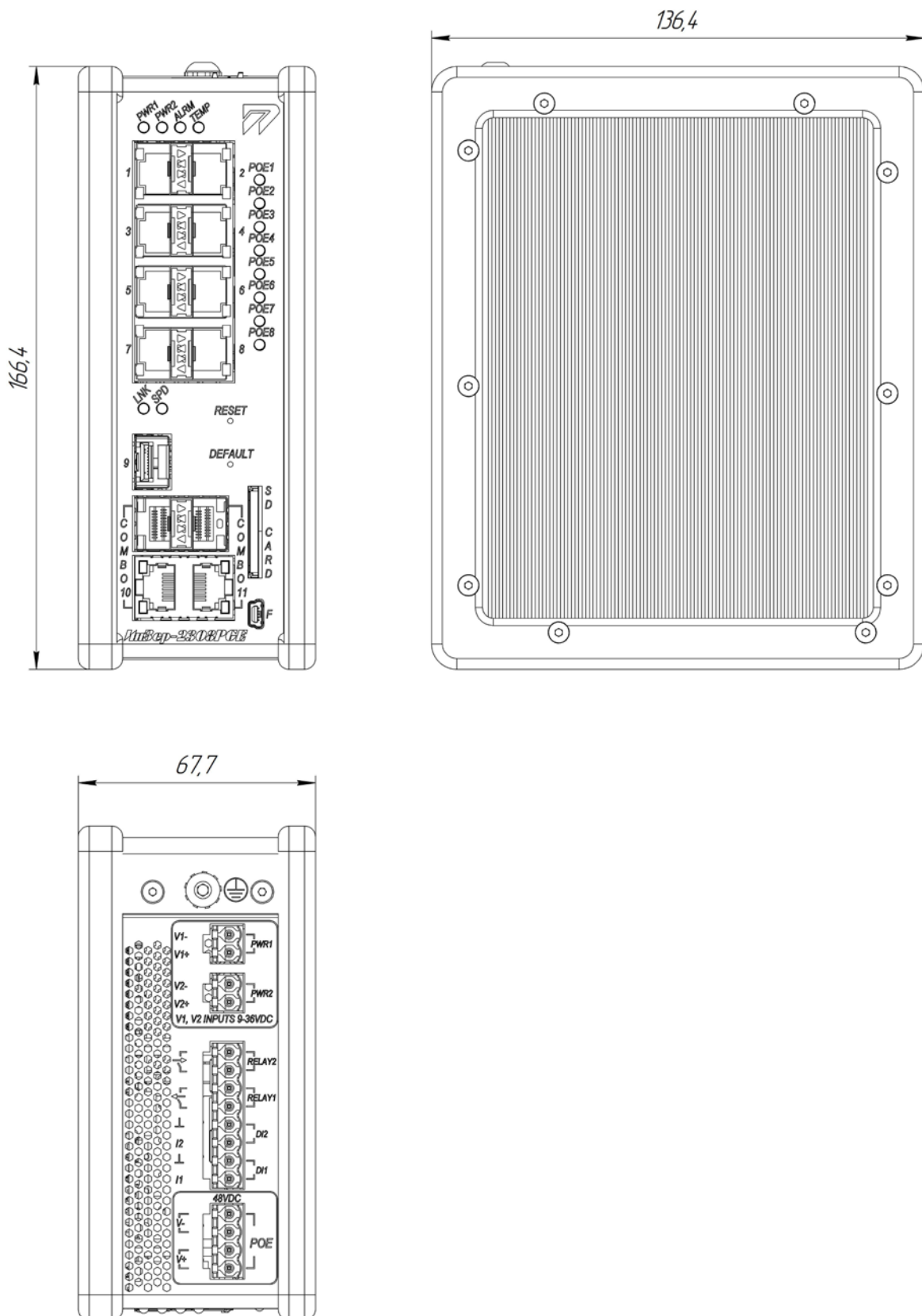
Рисунок А.1 – Габаритные и установочные размеры коммутатора
