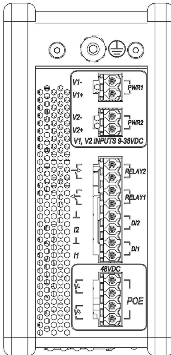
Рисунок Б.2 – Внешний вид верхней панели коммутатора
