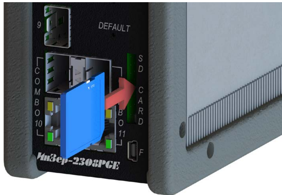
Рисунок 11 – Установка карты памяти в коммутатор
