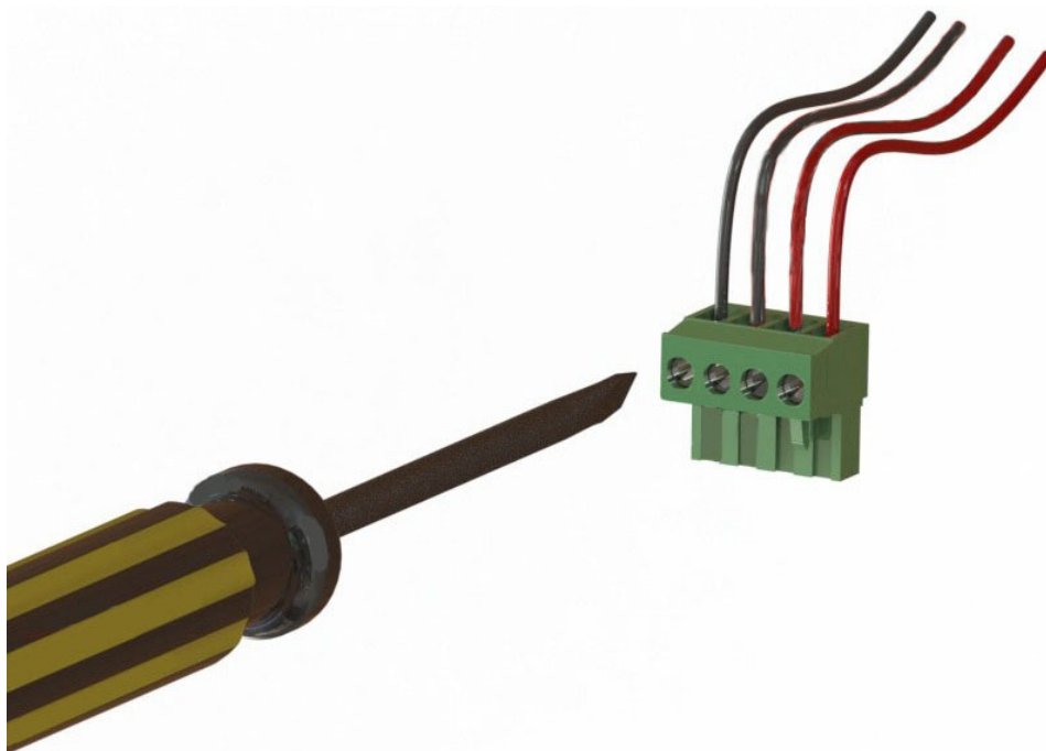
Рисунок 20 – Подключение проводов к ответной части разъема питания PoE
