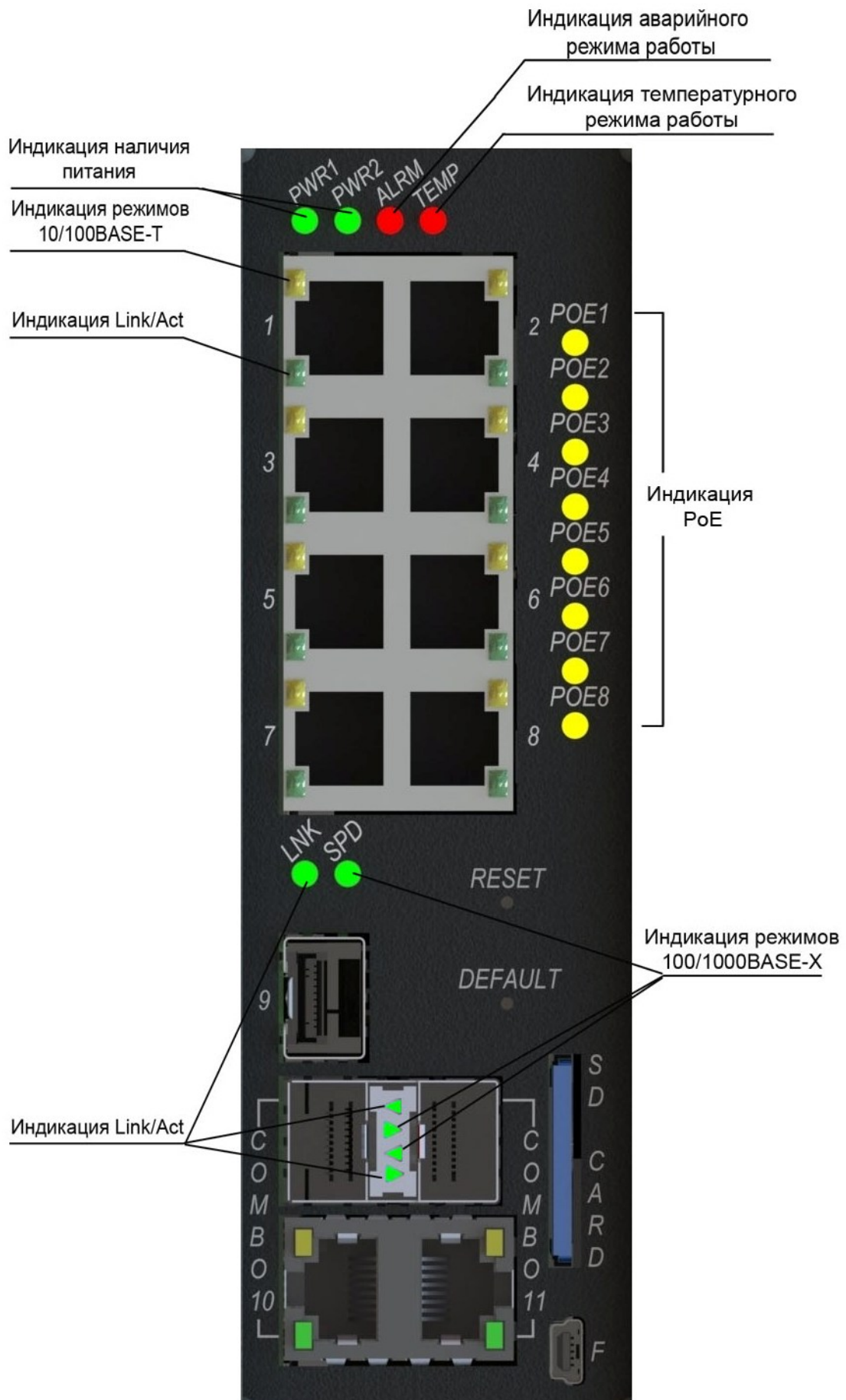
Рисунок 22 – Вид лицевой панели коммутатора ИнЗер-2xxx
