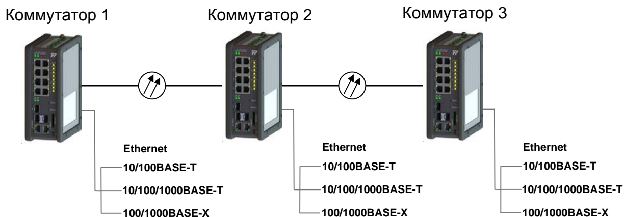
Рисунок 3 – Включение коммутаторов в линейную топологию
