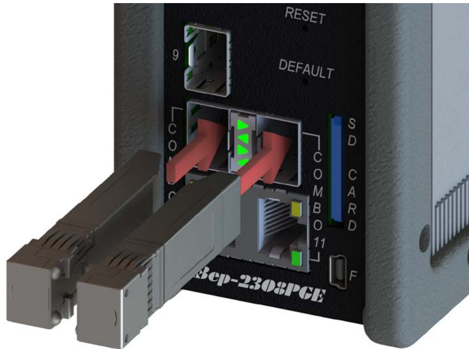
Рисунок 14 – Установка SFP-модулей в разъемы SFP
