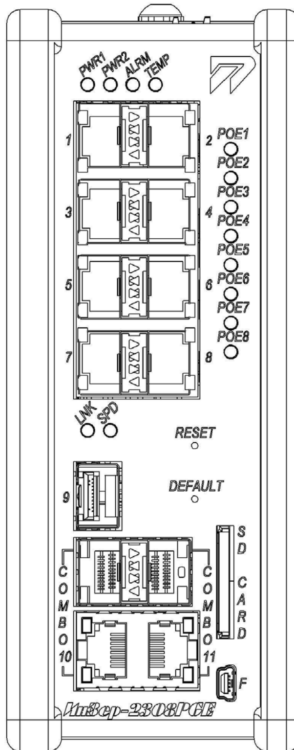
Рисунок Б.1 – Внешний вид лицевой панели коммутатора
