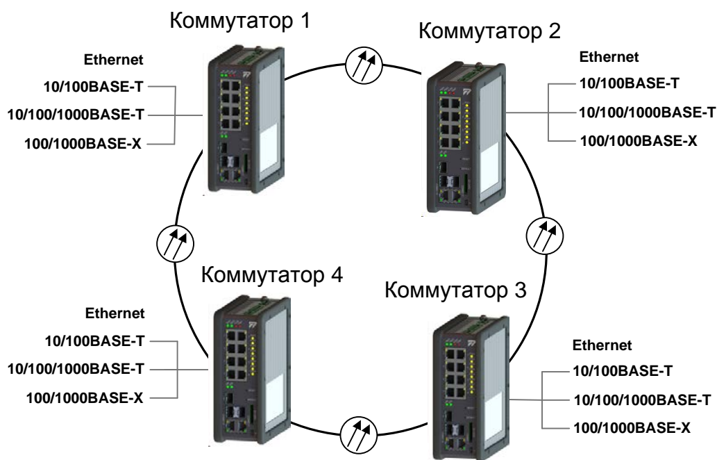
Рисунок 2 – Включение коммутаторов в кольцевую топологию
