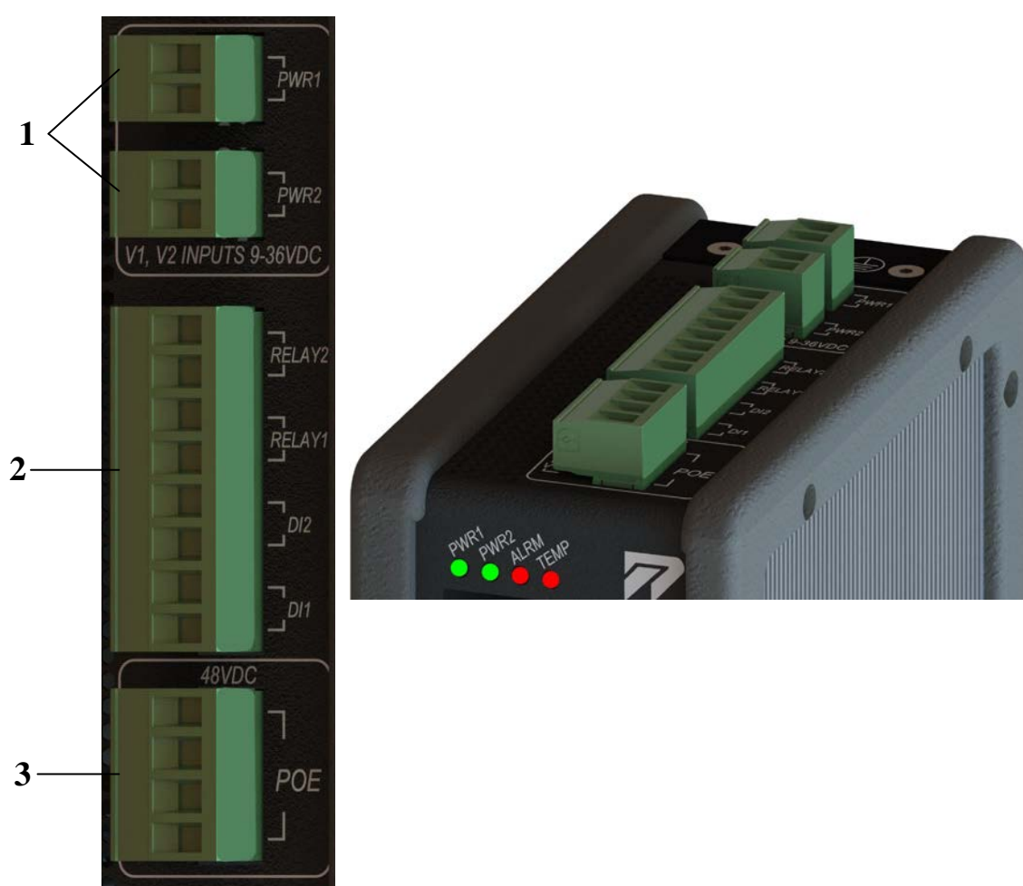
1 – разъемы питания; 2 – разъем «сухие контакты»; 3 – разъем питания PoE (только для коммутаторов с поддержкой PoE)
